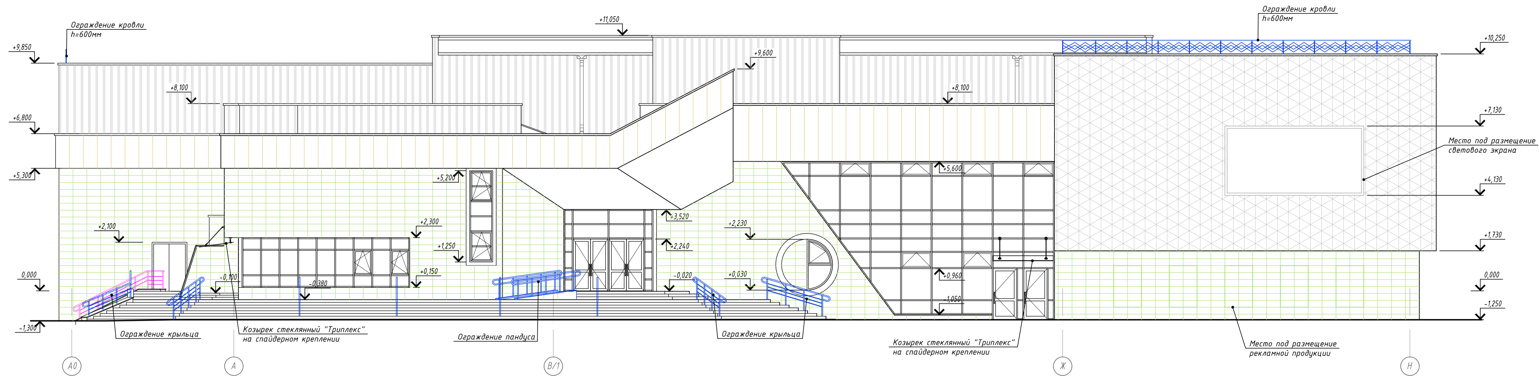
Фасад в осях А0-Н
