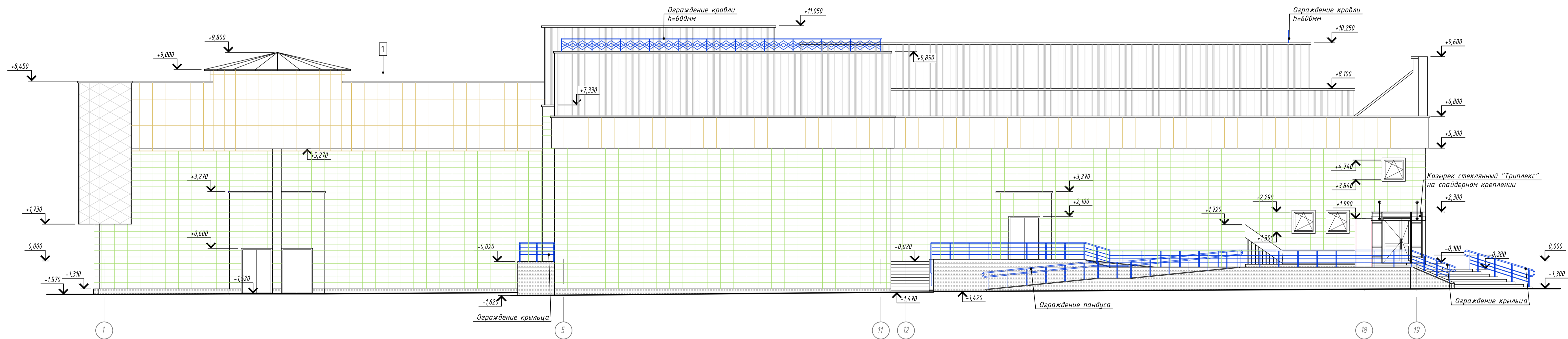
Фасад в осях 1-19
